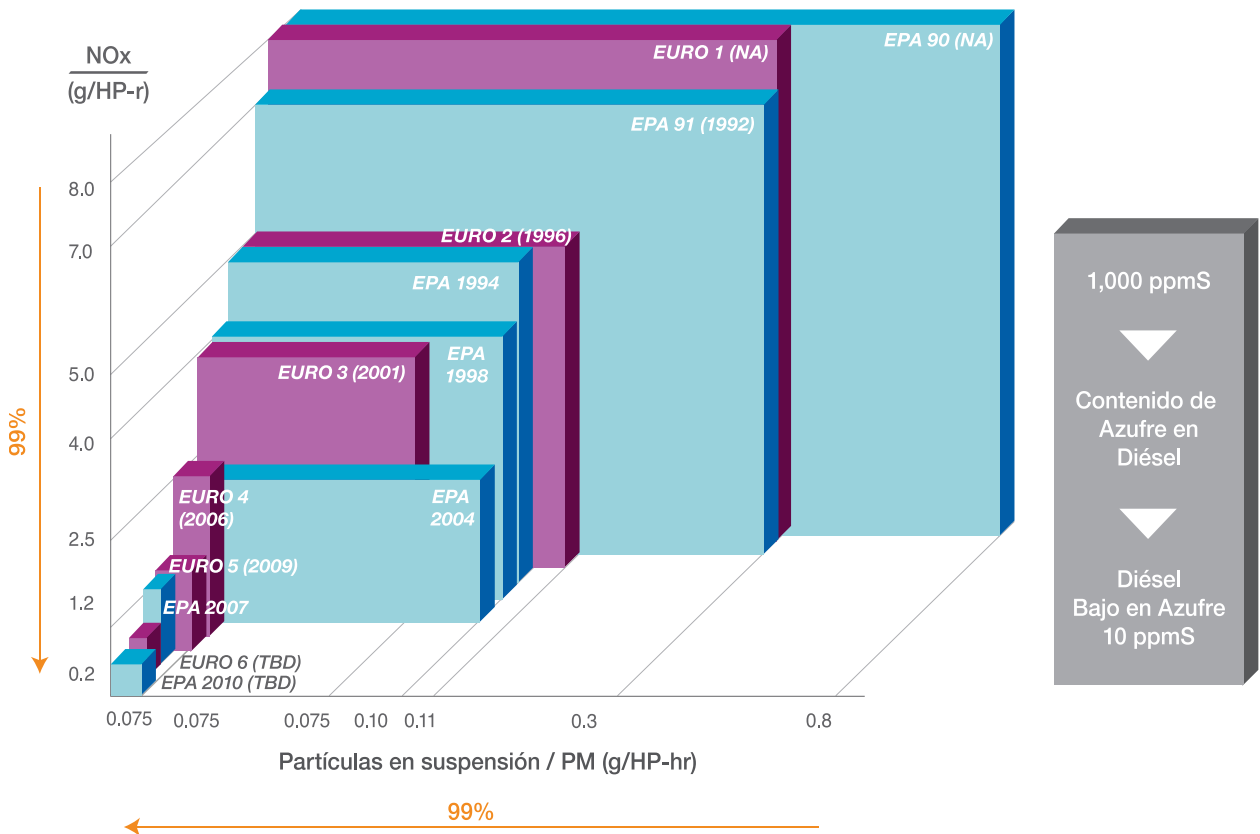
Imagen 3 Cantidad de emisiones de las normativas EPA y EURO.
