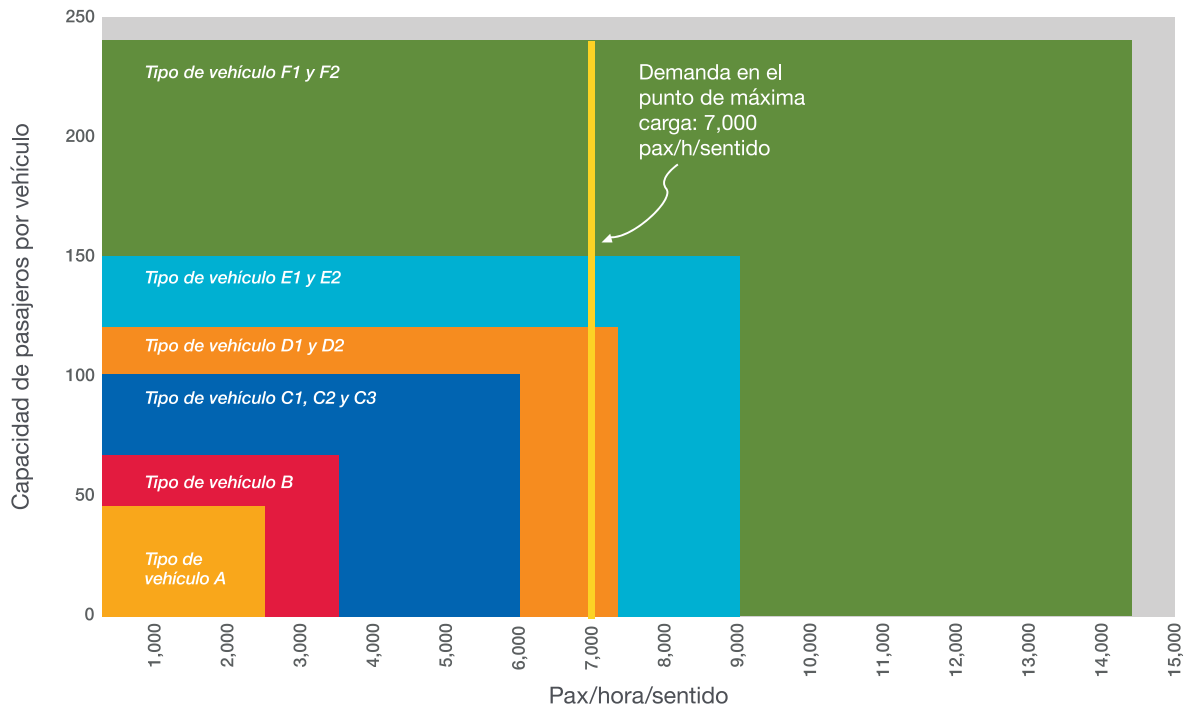
Gráfica 7 Tipo de unidad por capacidad en HMD y Demanda del proyecto (caso 1).
