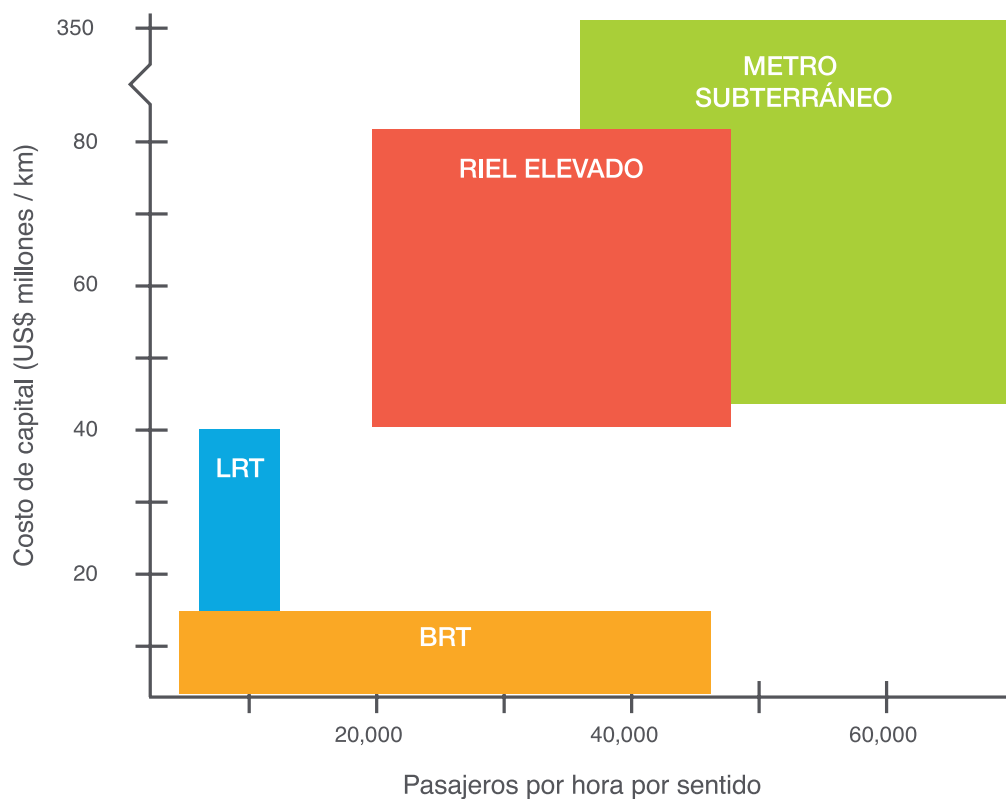
Gráfica 4 Tecnología a emplear de acuerdo con la demanda y el monto de la inversión.
