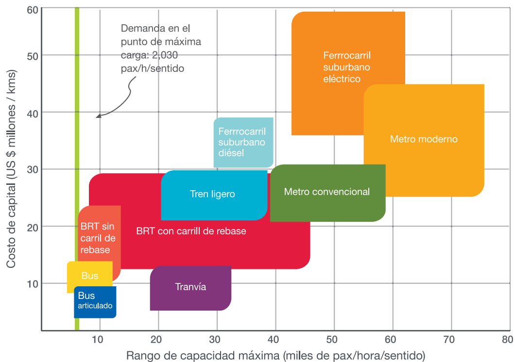
Gráfica 8 Tecnología, velocidad y demanda del proyecto (caso 2).
