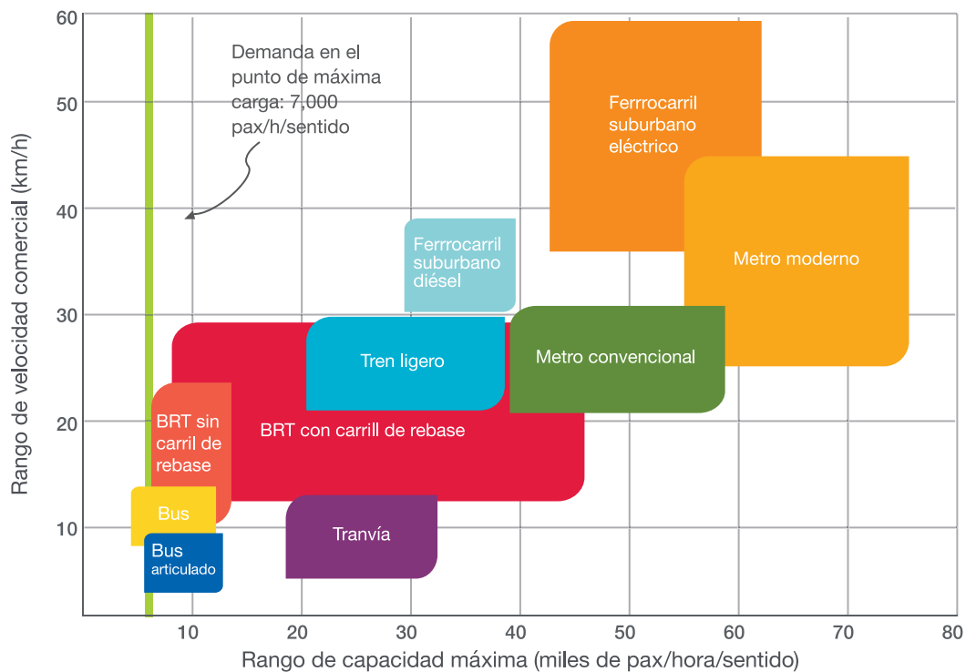
Gráfica 6 Tecnología, velocidad y demanda del proyecto (caso 1).
