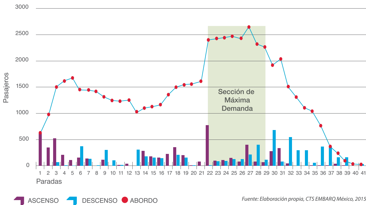
Gráfica 1 Ejemplo de polígono de carga (sección de máxima demanda).
