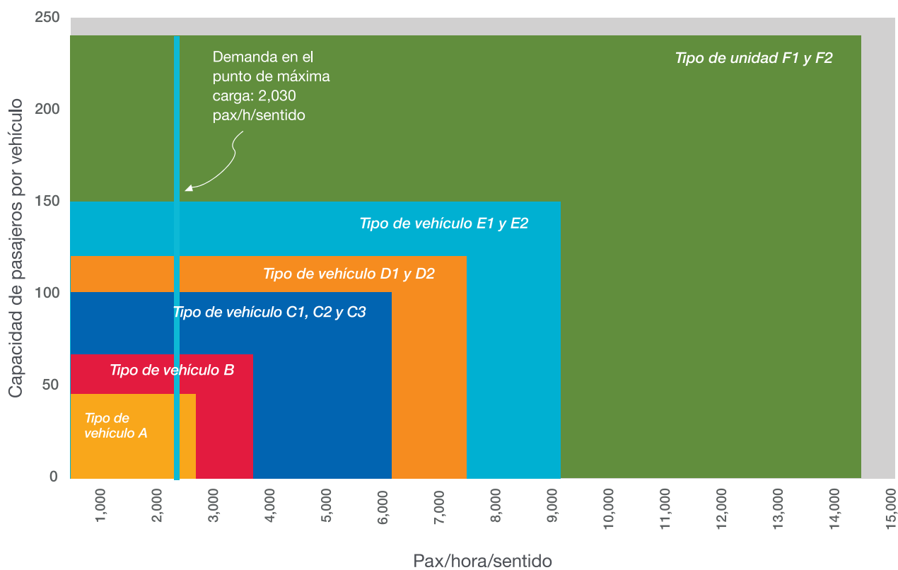
Gráfica 9 Tipo de unidad por capacidad en HMD y demanda del proyecto (caso 2).
