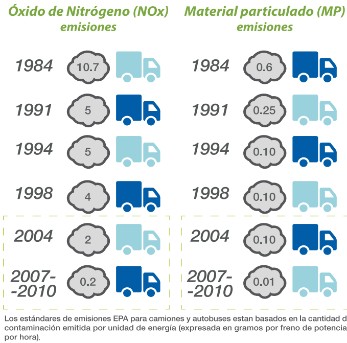
Imagen 2 Emisiones de óxidos de nitrógeno y material particulado por cada unidad de energía y su evolución a lo largo del tiempo, desde 1984 hasta el año 2010.
